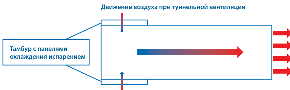
Рис. 39: Движение воздуха при туннельной вентиляции.
