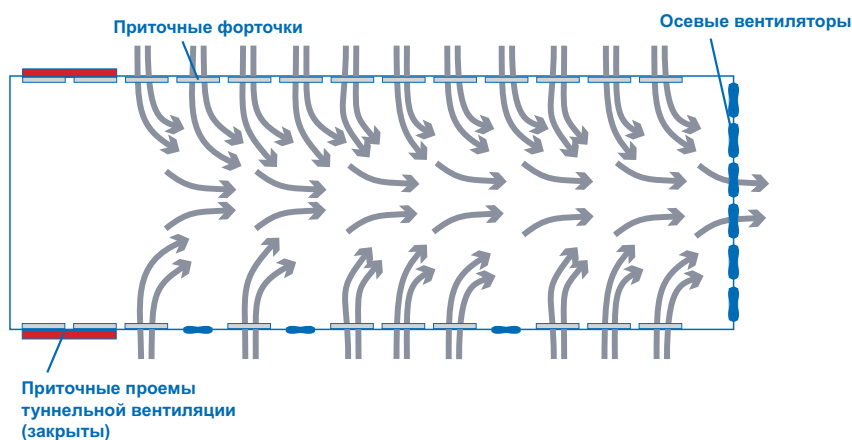
Рис. 38: Движение воздуха в птичнике при переходной вентиляции.
