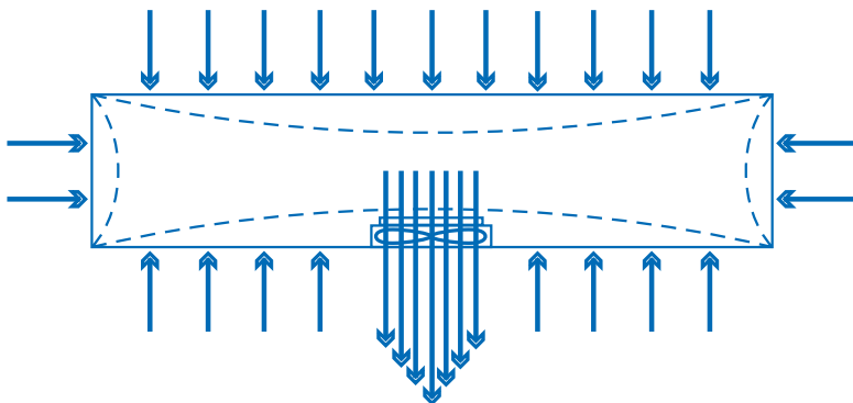
Рис. 31: Схема, иллюстрирующая движение воздуха через приточные форточки при отрицательном давлении.
