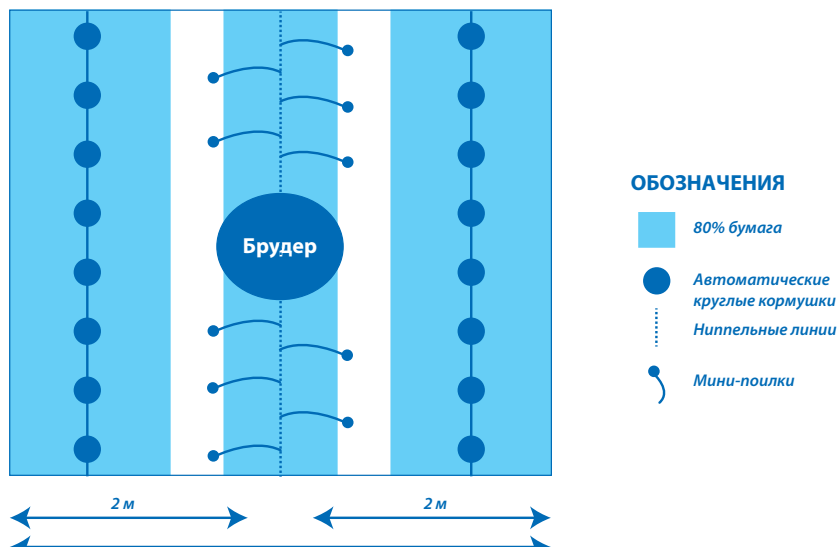
Рис. 9: Типичная планировка птичника при точечном выращивании (1000 голов).
