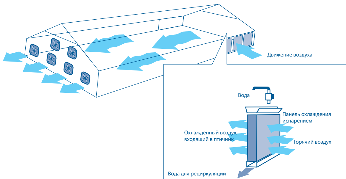
Рис. 44: Работа панелей испарения с туннельной вентиляцией.
