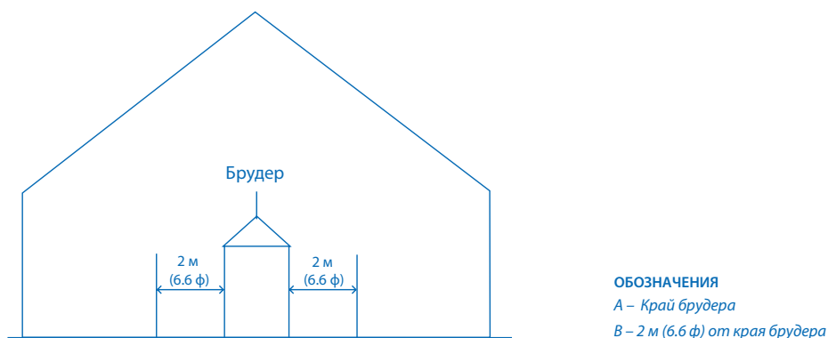
Рис. 10: Точечное выращивание - температурные зоны.
